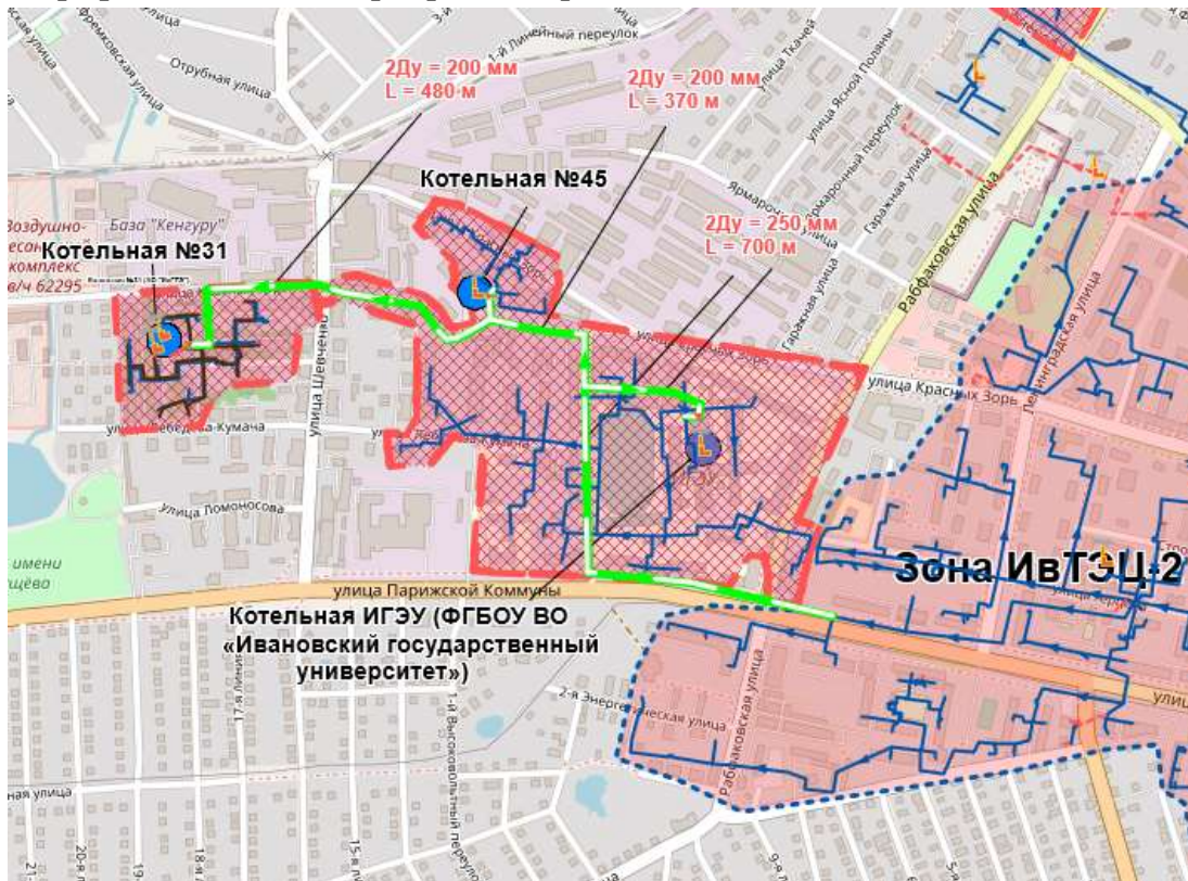
Рис. 4.47. Мероприятия переключения потребителей котельных №31, №45, ИГЭУ на ИВГЭЦ-2 со строительством участков сети и трех ЦТП
