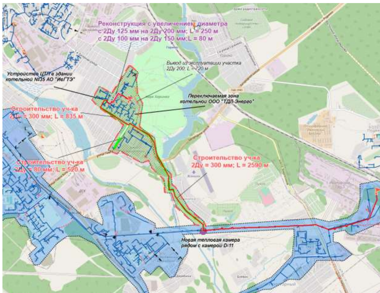
Рис. 4.30. Путь для построения пьезометрического графика участка тепловой сети от ИвТЭЦ-3 в зону котельной ООО «ТДЛ-Энерго» до потребителя по адресу ул. 2-я Лагерная 53 (Сценарий 3)
