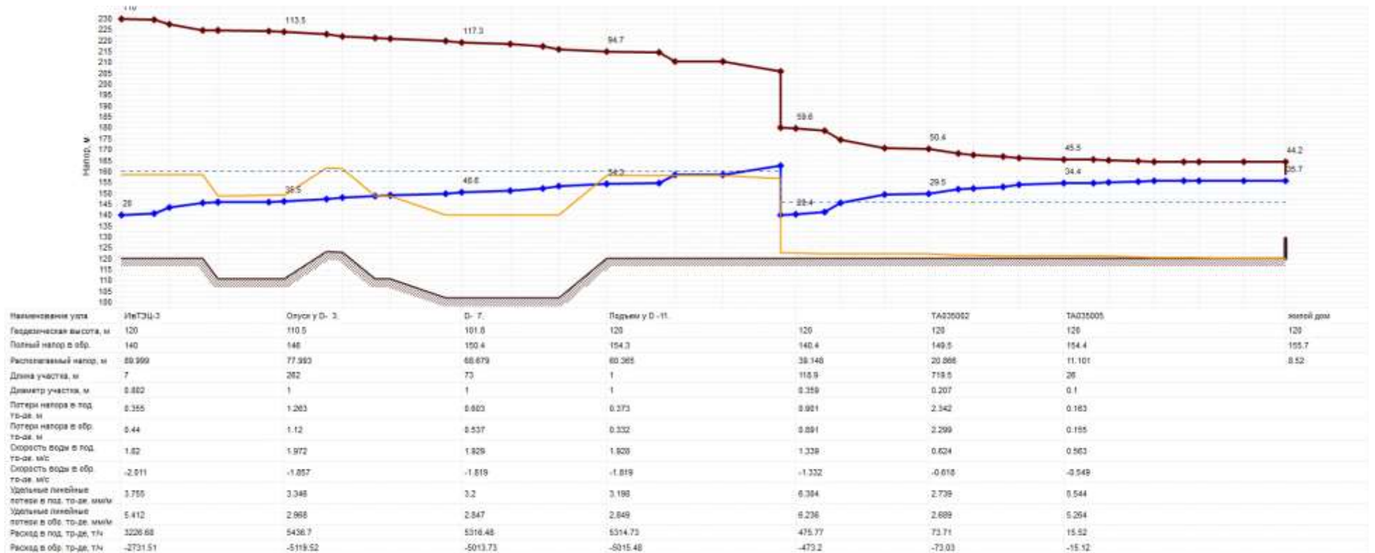
Рис. 4.34. Пьезометрический график участка тепловой сети от ИвТЭЦ-3 в зону котельной ООО «ТДЛ-Энерго» до потребителя по адресу ул. 2-я Лагерная 53 (Сценарий 4)
