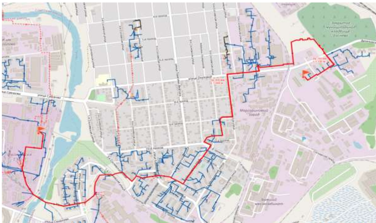
Рис. 4.2. Путь для построения пьезометрического графика участка тепловой сети от ИвТЭЦ-2 в зону действия котельной по адресу г. Иваново, ул. Окуловой, 74Б
