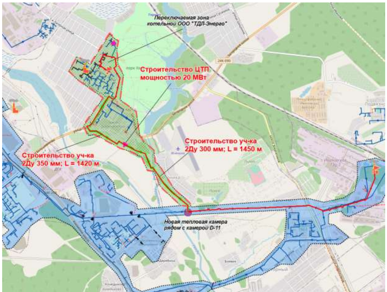
Рис. 4.33. Путь для построения пьезометрического графика участка тепловой сети от ИвТЭЦ-3 в зону котельной ООО «ТДЛ-Энерго» до потребителя по адресу ул. 2-я Лагерная 53 (Сценарий 4)
