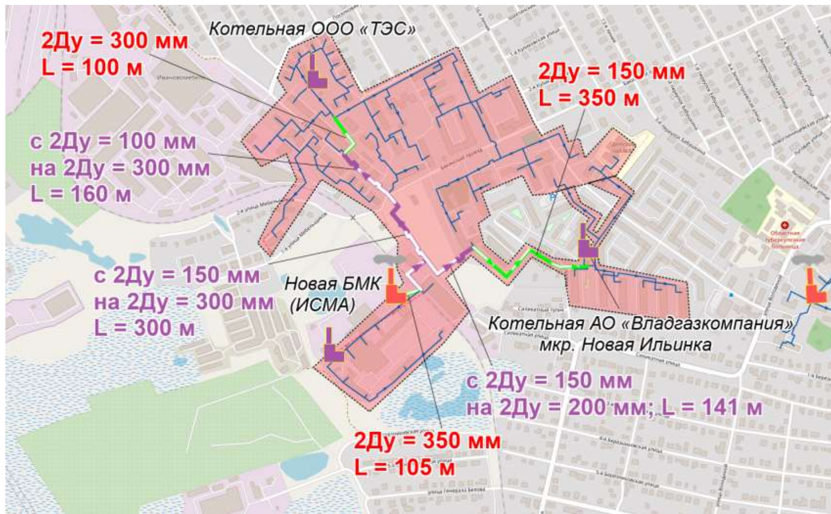
Рис. 4.18. Перспективные зоны источников тепловой энергии после переключения котельной ООО «Система Альфа» и АО «Владгазкомпания» (мкр. Новая Ильинка) на новую БМК по Сценарию 4
