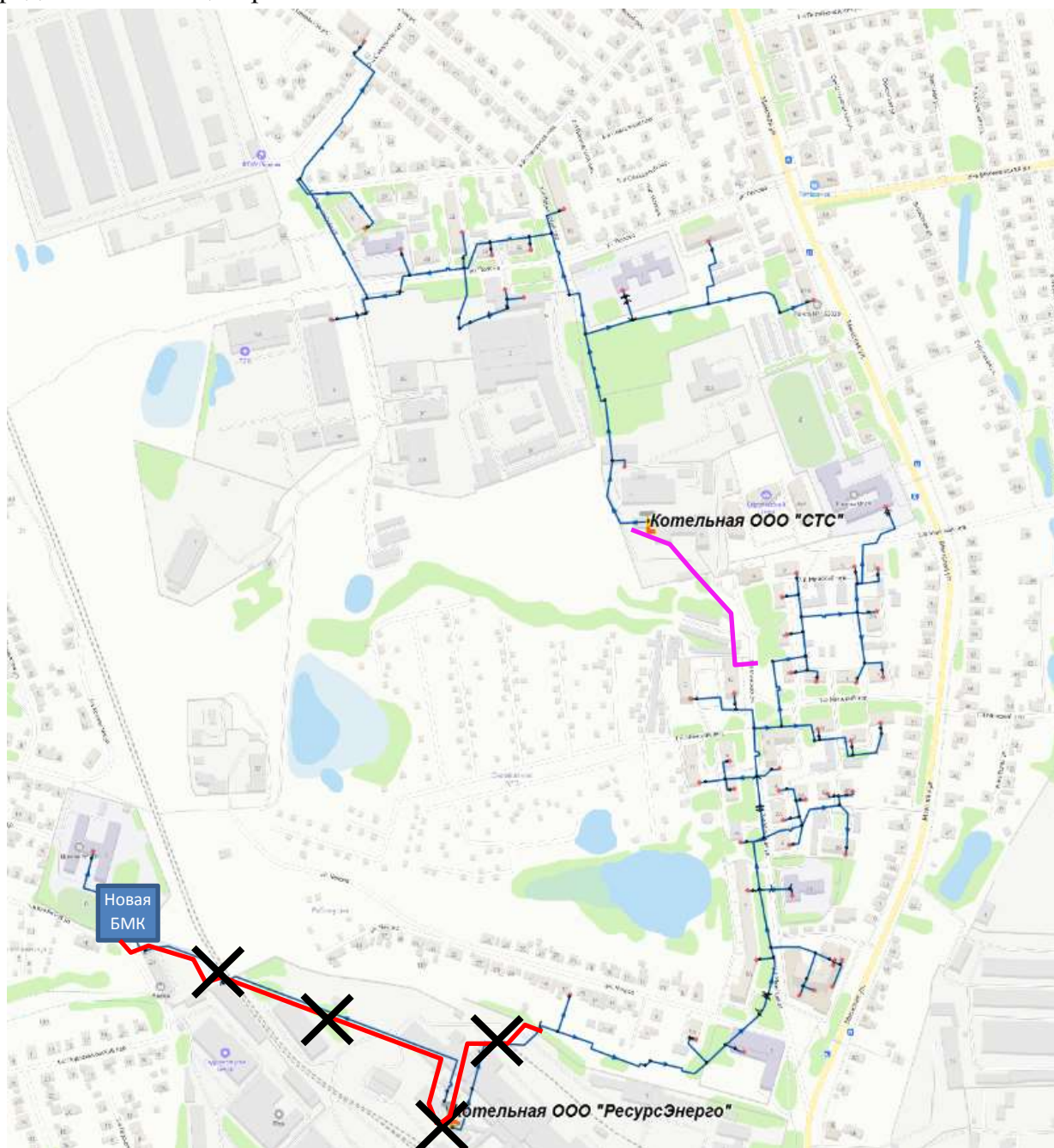
Рис. 4.54. Перспективная зона после переключения потребителей котельной ООО «Ресурс-Энерго» на котельную ООО «СТС»
