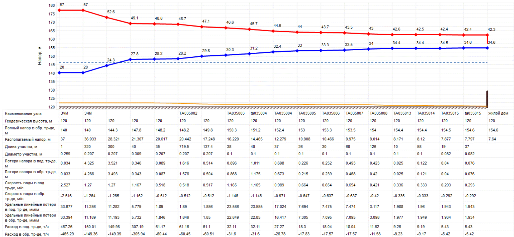
Рис. 4.25. Пьезометрический график участка тепловой сети от котельной ООО «ТДЛ-Энерго» до потребителя по адресу ул. 2-я Лагерная 53 (Существующее положение)
