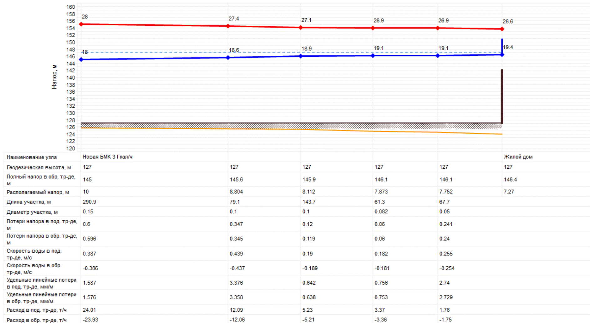
Рис. 4.41. Пьезометрический график участка тепловой сети от новой БМК мощностью 3,0 Гкал/ч в зону котельной № 42 (ФГБУ «ЦЖКУ» Минобороны России) до потребителя по адресу ул. Автодорожская, 10 (Сценарий 1)
