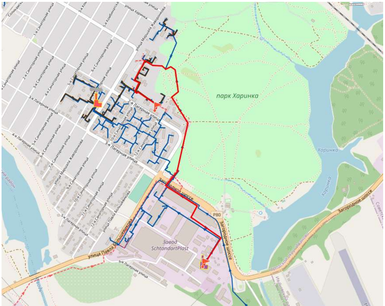
Рис. 4.24. Путь для построения пьезометрического графика участка тепловой сети от котельной ООО «ТДЛ-Энерго» до потребителя по адресу ул. 2-я Лагерная 53 (Существующее положение)
