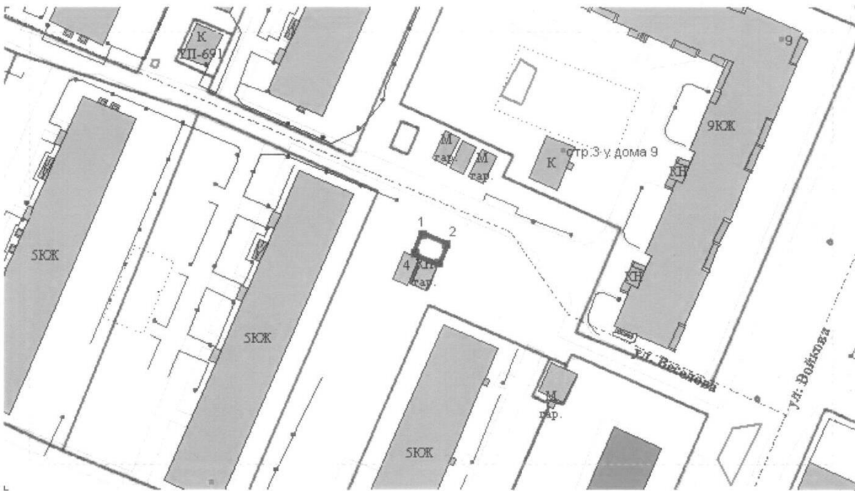
Графическая схема № 13 размещения гаража, являющегося некапитальным сооружением, площадью 24 кв. м, у дома 9 по улице Гагарина в городе Иваново
